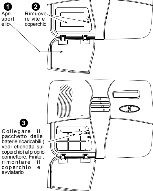
Figura 10. Sostituzione delle batterie
