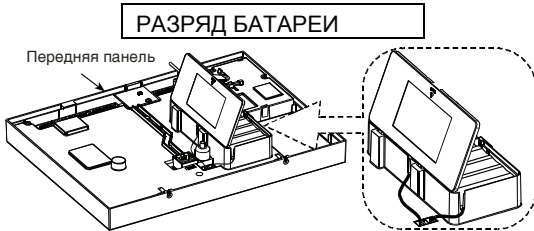
Рисунок 10. Замена аккумулятора
