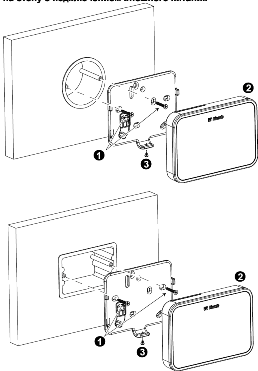
Рисунок 4b – Монтаж на стену с внешним питанием
