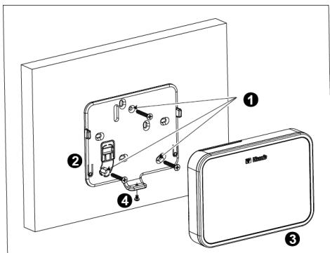
Рисунок 4а – Монтаж на стену
