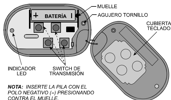
Figura 2. Vista interior con la tapa quitada
