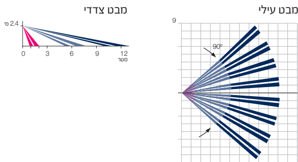
TOWER-20AM PG2 זווית רחבה
